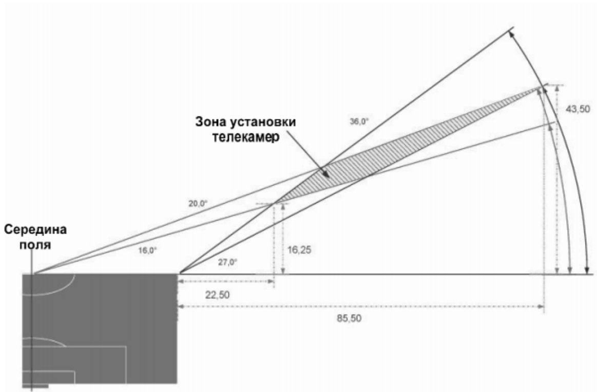
Схема розміщення телевізійних камер офіційного мовника уздовж бічної лінії поля з розрахунком згідно рекомендацій UEFA
